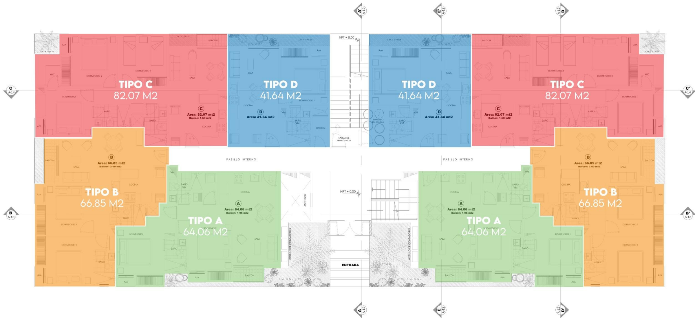
PLANTA ARQUITECTURA NIVEL 1 (N+0.00)
